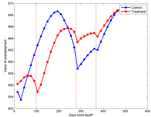
(d) Value of Unemployment, Reference-Dependent model
