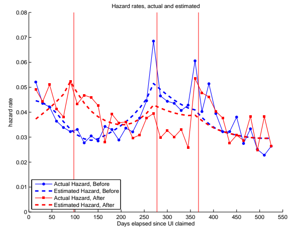
(d) Ref. Dep. Model, no heterogeneity, estimated \beta
