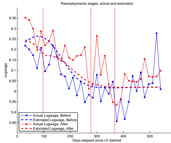
(d) Reemployment Wage in Ref. Dep. Model
