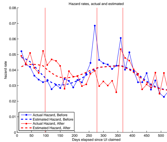
(d) Heterogeneity in Search Cost Elasticity
