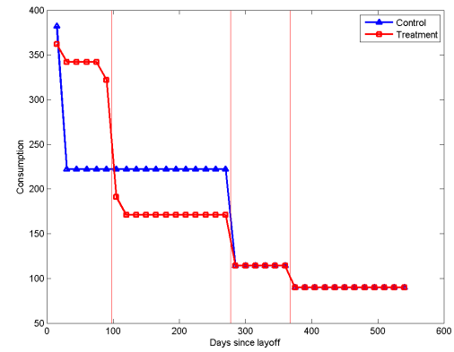
(d) Consumption, Reference-Dependent model
