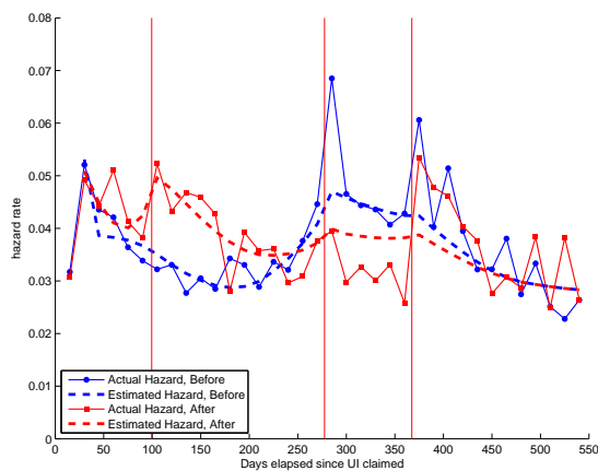
(d) Ref. Dep. Model: Estimation without Spikes
